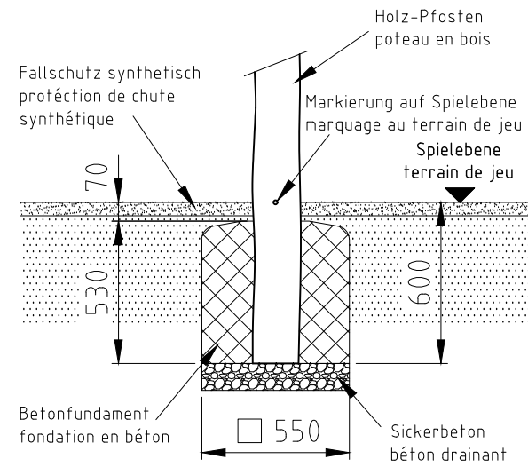
Fundament F01
