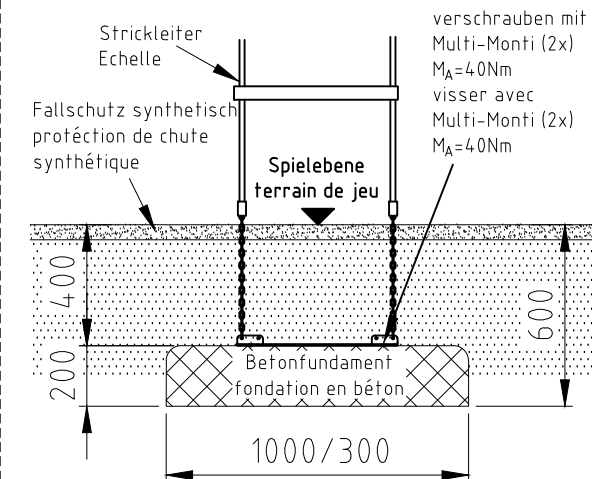
Fundament F15
