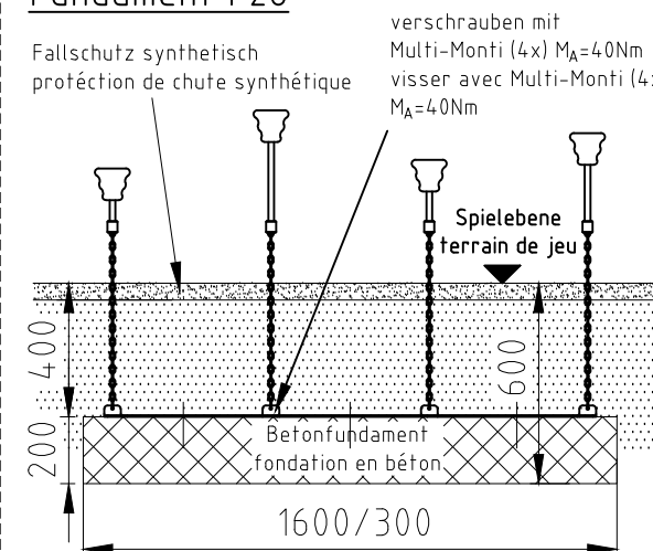
Fundament F26
