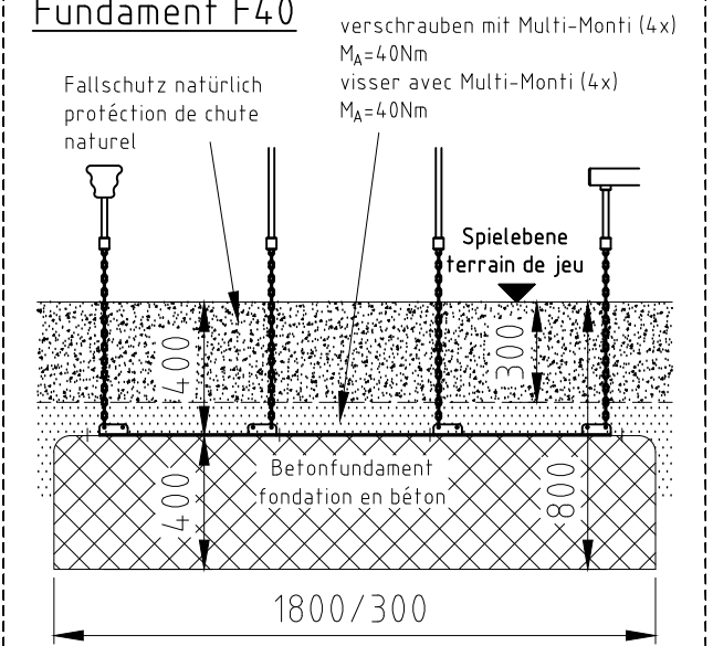
Fundament F40
