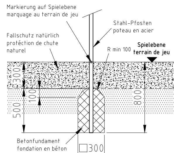
Fundament F20
