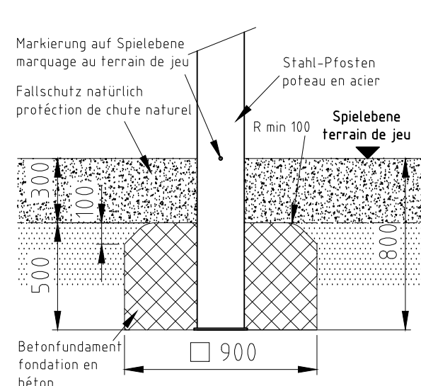
Fundament F20
