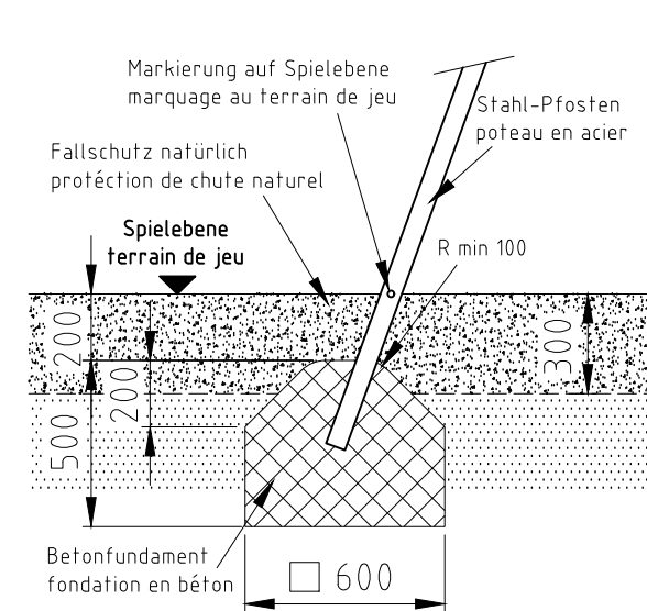
Fundament F18
