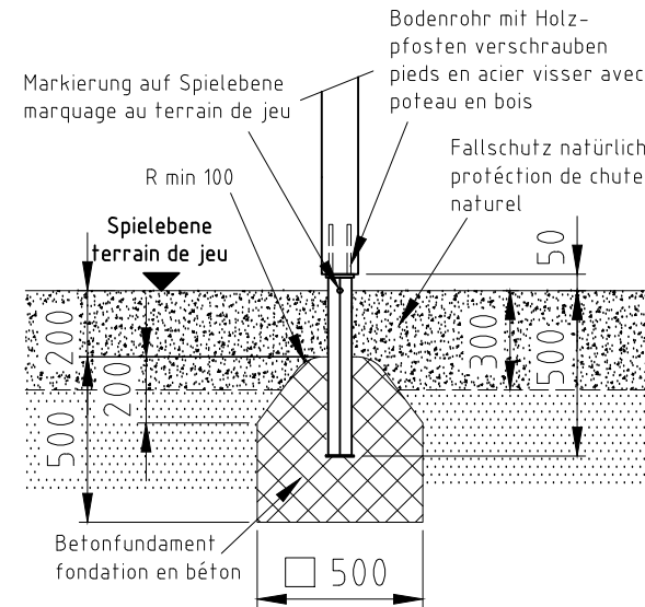
Fundament F01
