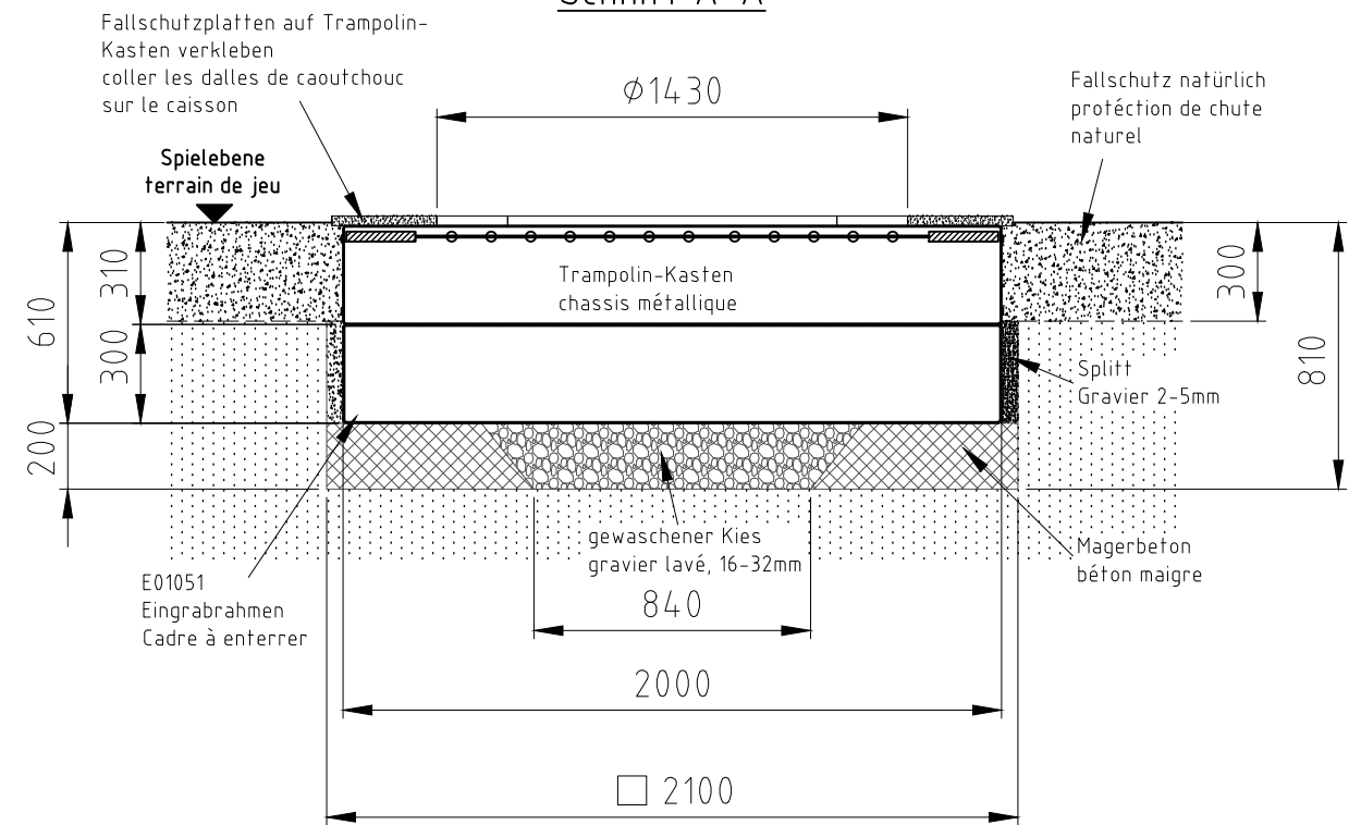
Schnitt A-A
